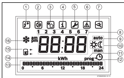
Fig. 21 Display
