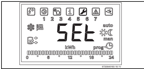
Fig. 29 "Set" function
